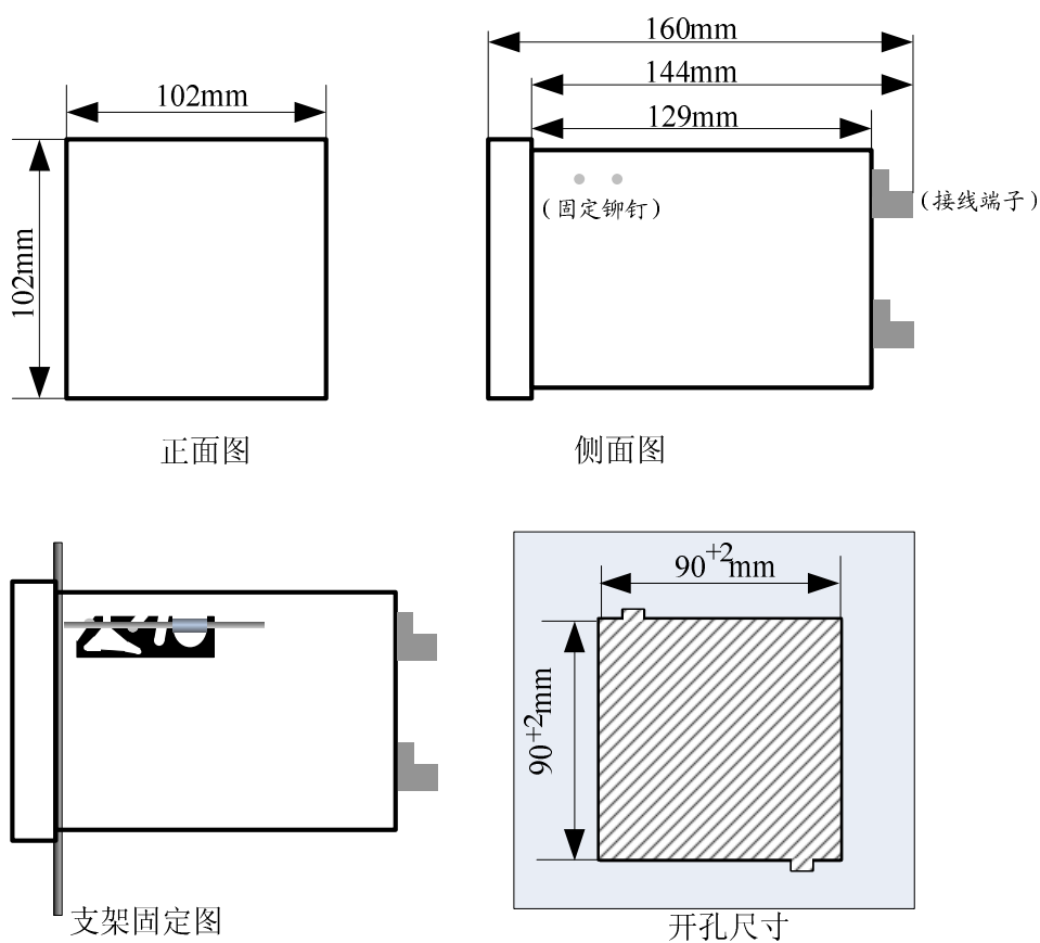
安装示意图
